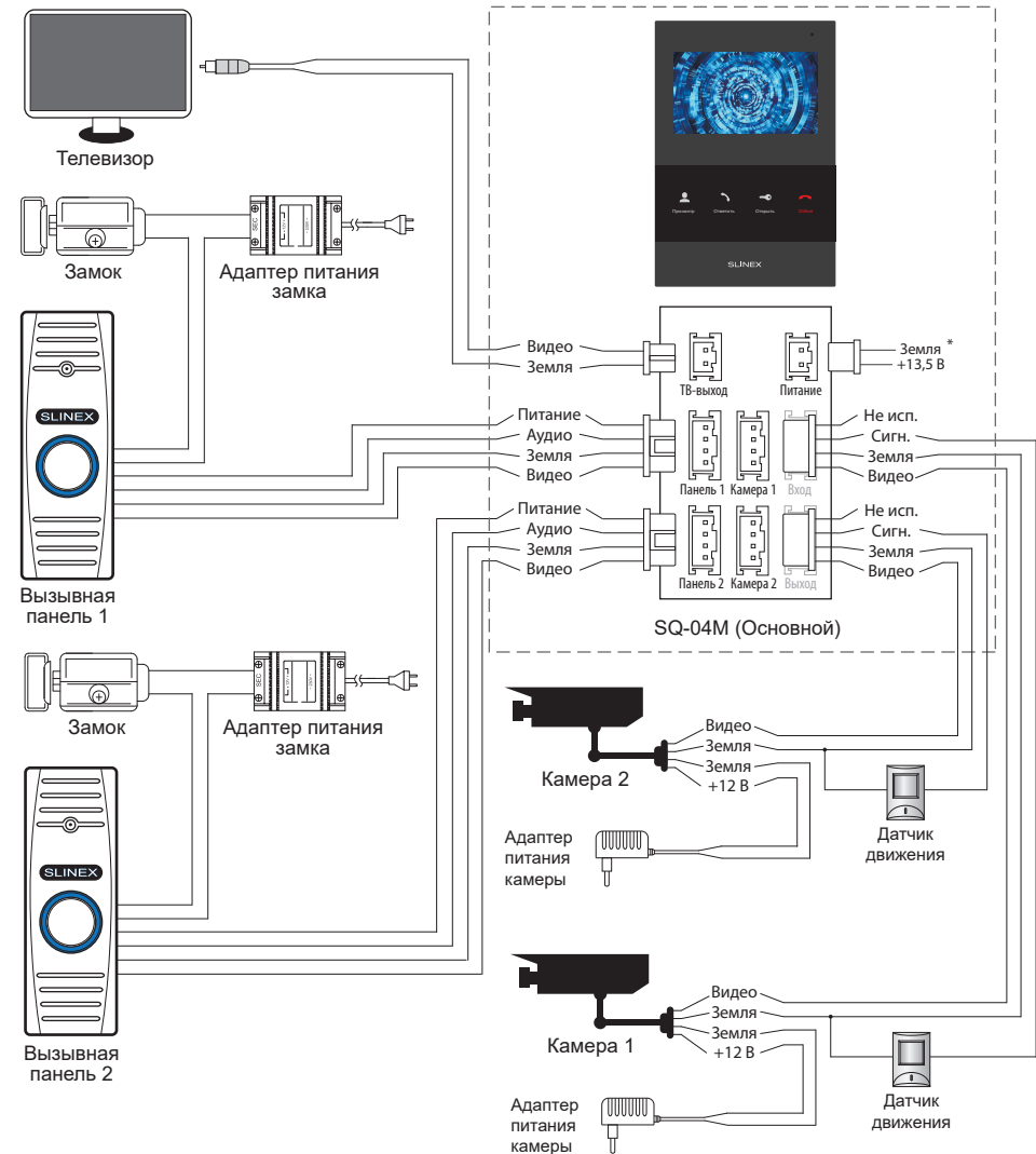
Схема 1. Подключение вызывных панелей, камер и телевизора к домофону SQ-04M
